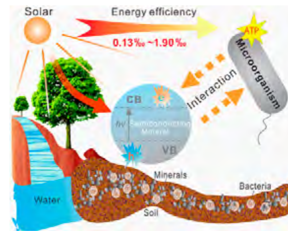
自然界中半导体矿物日光催化作用促进“光电微生物”生长代谢示意图
